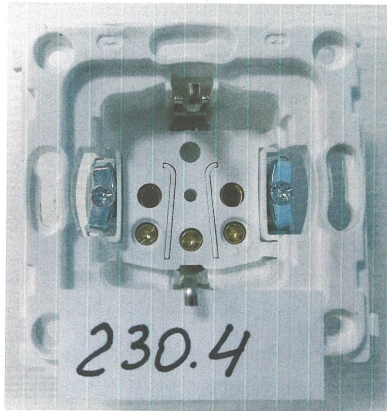
Внешний вид образца испытаний
