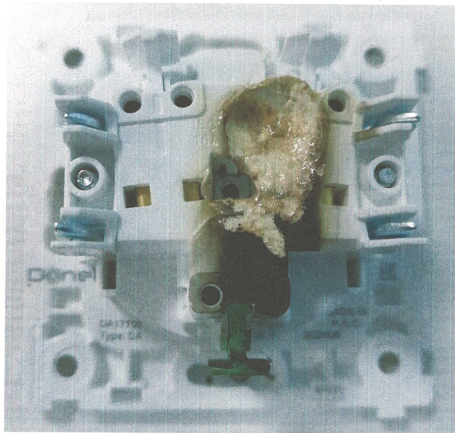
Состояние образца после испытаний
