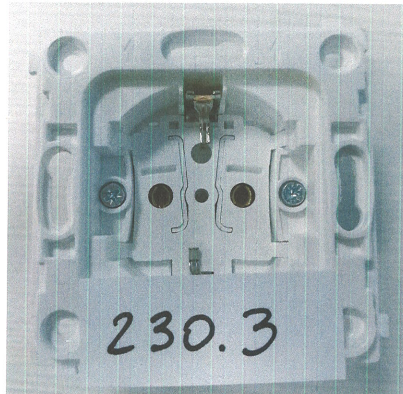
Внешний вид образца испытаний
